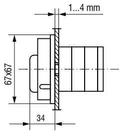
Type D (RC-40)
