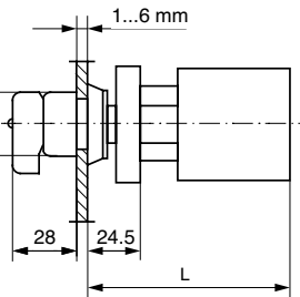
Type B (RC-40)
