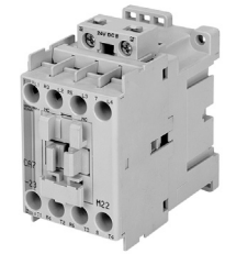
CA7-23E-M22-24E contactor
